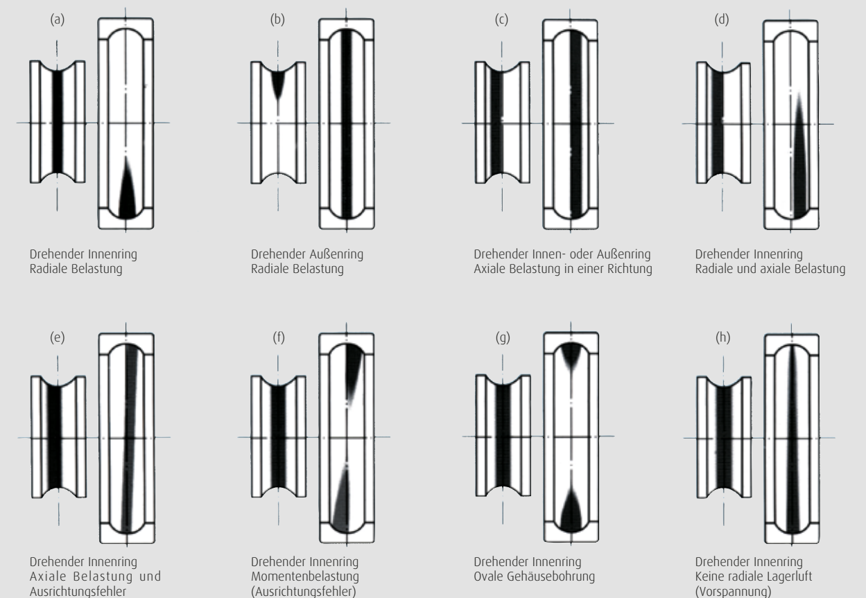
Abb. 3 Typische Laufspuren an Rillenkugellagern
