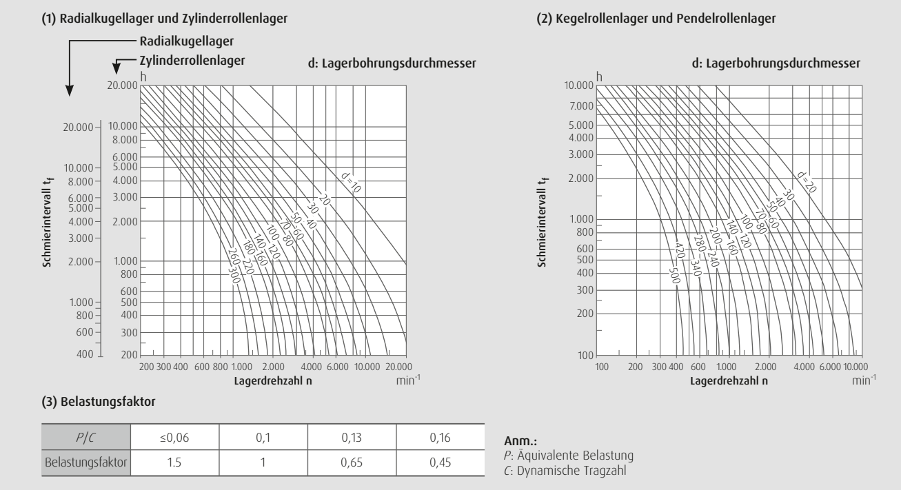
Abb. 2 Schmierintervalle
