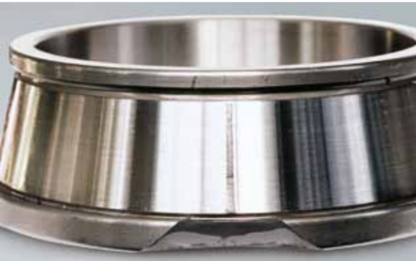
Foto 5.2 Bauteil: Innenring eines Kegelrollenlagers Symptom: Bruch des Innenringbords Ursache: Starke Stöße während des Einbaus
