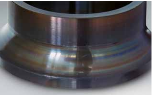
Foto 18.1 Bauteil: Innenring eines Schrägkugellagers Symptom: Blau- oder Lilafärbung der Laufbahn Ursache: Wärmeentwicklung aufgrund von Mangelschmierung
