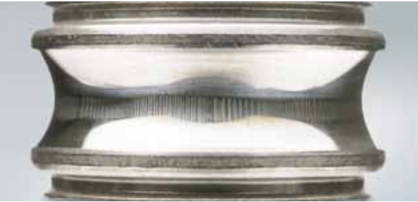
Foto 15.5 Bauteil: Innenring eines Rillenkugellagers Symptom: Riffelungen an der Laufbahn (Durchgang von hochfrequentem Strom)
