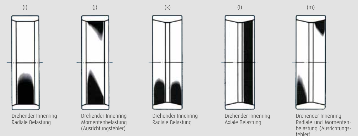
Abb. 4 Typische Laufspuren an Rollenlagern
