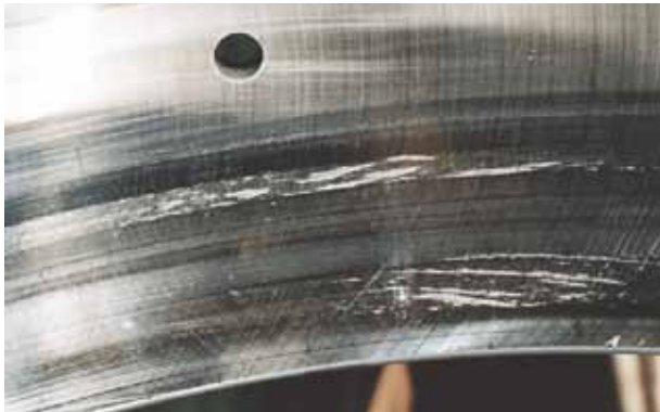
Foto 4.6 Bauteil: Außenring zu Foto 4.5 Symptom: Teilweise Anschmierungen am Umfang der Laufbahn Ursache: Mangelschmierung
