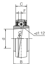
UK2
