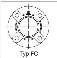
Typ FC
