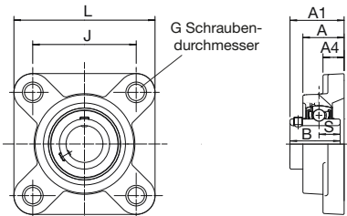
Reihe PSF/LP99
