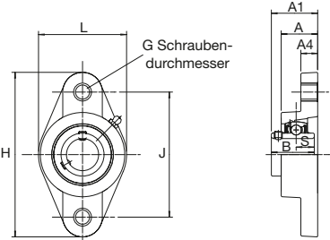
Reihe PSFT
