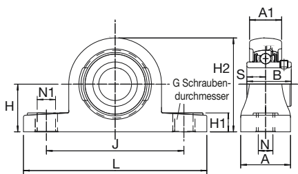
Reihe PNP/LP99
