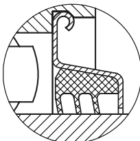
Typ L3 Dreifachlippendichtung
