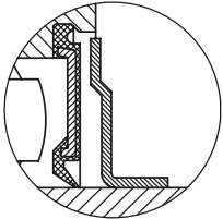
Typ SL Doppellippendichtung
