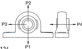
Reihe PNP
