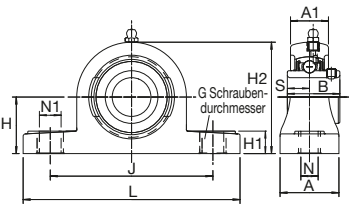
Reihe PNP
