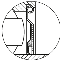
Typ H mit Stahlblecheinsatz
