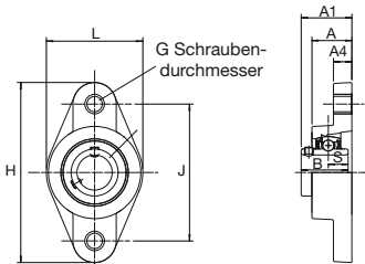
Reihe PSFT/LP99
