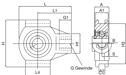
Reihe PST/LP99
