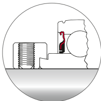
Exzenterring
