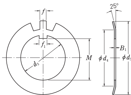
Gerade Laschen
