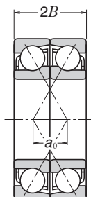
X-Anordnung DF
