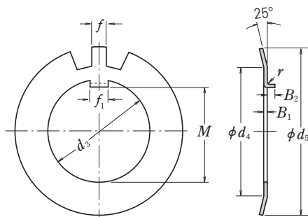
Gebogene Laschen
