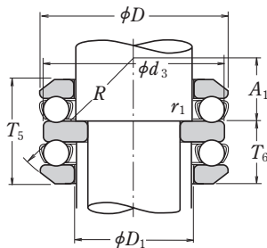
Mit kugeligter Auflagefläche
