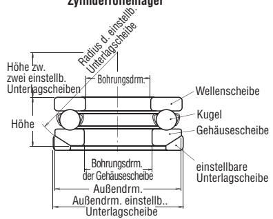
Einseitig wirkendes Axialkugellager
