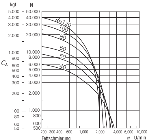
Abb. 5.13 Zulässige Axiallast für Zylinderrollenlager Für Lager der Durchmesserreihe 3 ( k=1,0 ), die unter ständiger Belastung betrieben und mit Fett oder Öl geschmiert werden.
