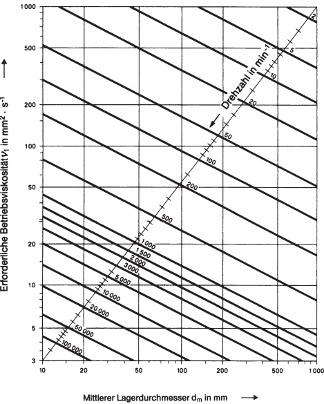
Abb 12.12 Durchmesser- und drehzahlabhängige Bezugsviskosität
