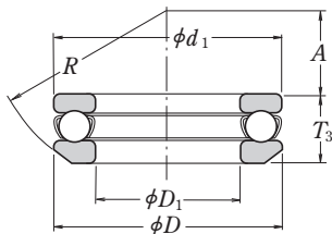
Mit kugeliger Auflagefläche
