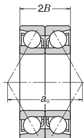
O-Anordnung DB
