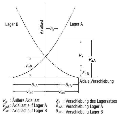
Abb. 10.4 Axiale Verschiebung bei starrer Vorspannung
