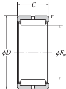
Ohne Innenring RNA
