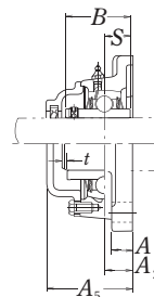
Gusseisen, Ausführung mit Staubabdeckung
