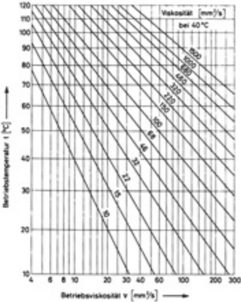
Abb 12.11 Viskositäts-Temperatur-Verhalten von Schmierölen
