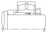
Abb. 14.4 Montage mit Spannhülse
