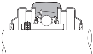
Abb. 2.2 Schutzkappe aus Stahlblech
