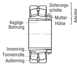
Pendelrollenlager
