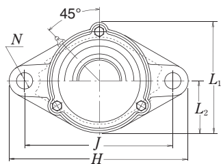
Gusseisen, Ausführung mit Staubabdeckung Offene Seiten Č-UCFL...D1 Geschlossene Seiten CM-UCFL...D1
