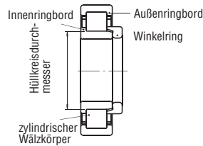
Zylinderrollenlager
