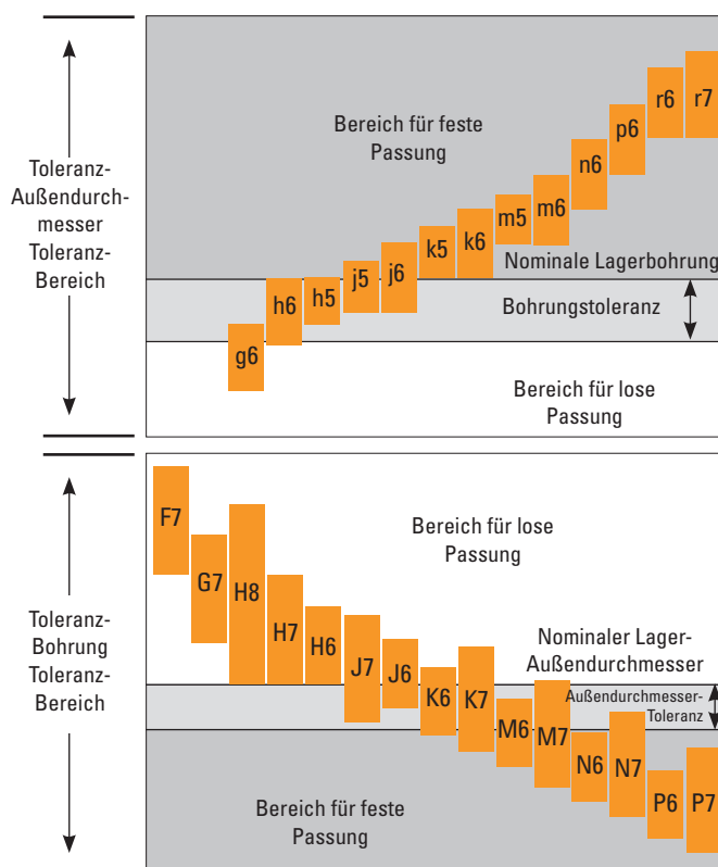
Abb. 5. Passungsauswahl für Welle und Gehäuse.
