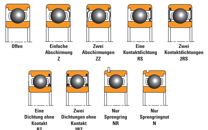
Abb. 4. Rillenkugellager-Varianten
