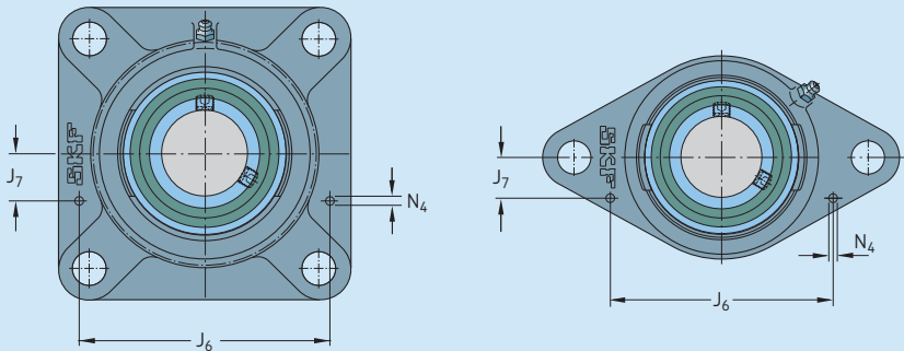
Abmessungen bei den Flanschlagereinheiten der Baureihen FY, FYJ
