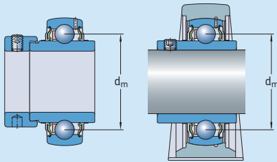
Mittlerer Lagerdurchmesser d_m
