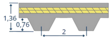
S2M
