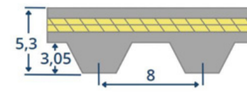
S8M
