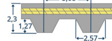
XL
