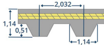
MXL
