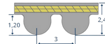
HTD 3M
